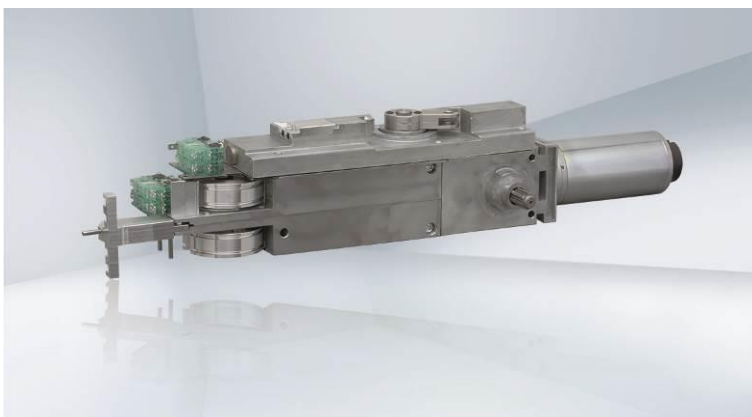
Bild 1: Der funktionsintegrierte Türantrieb von ebm-papst ZEITLAUF
