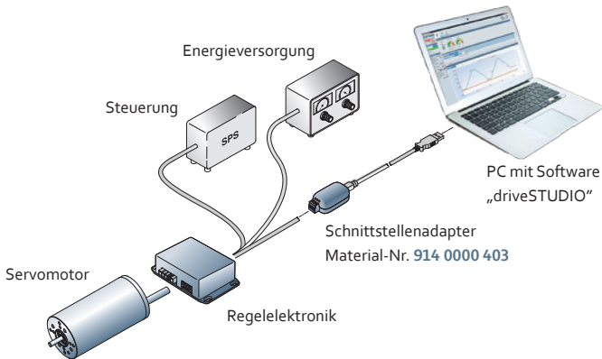
Anordnung Inbetriebnahme
