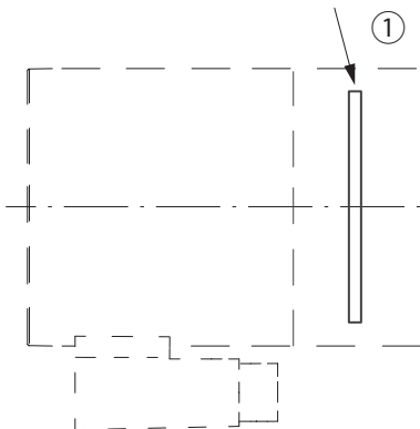
Abbildung mit integriertem Inkrementalgeber IEM 58 für ECI 63 K1
