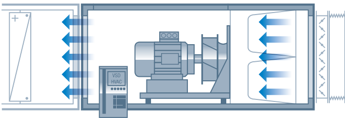
AC-Ventilatoren (AC-Standard-Motor mit Frequenzumrichter)
