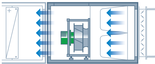
GreenTech EC-Ventilatoren
